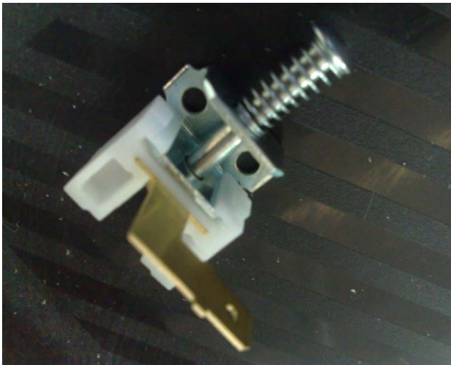
Inyección del cuerpo en POM, y montaje del muelle, faston y guía.
