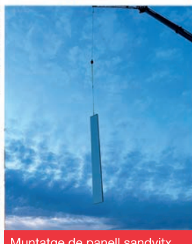
Muntatge de panell sandvitx
