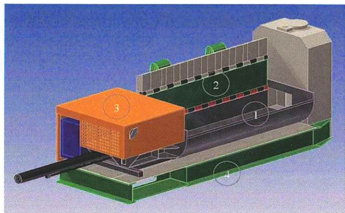
Caja de compresion conformada en "bañera"
