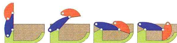
Caja de compresion conformada en "bañera"
