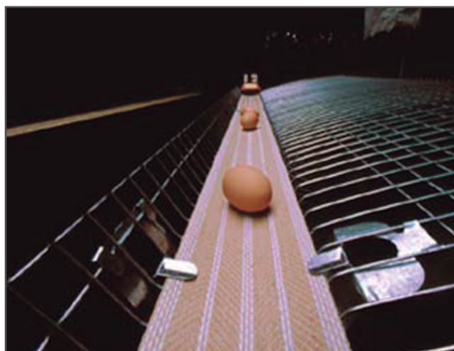
Bandas de yute y PP para la recogida de huevos . Se sirve en rollos, anchos y longitudes según cliente.
