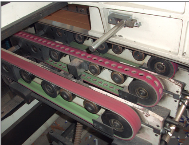
Correas planas con recubrimiento y/ o agujeros introdutoras de cartón.
